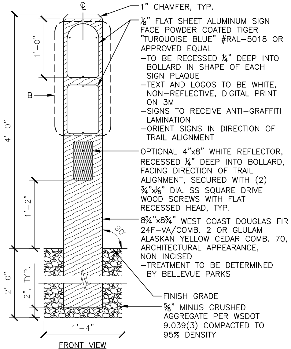
A-BOLLARD DETAIL
