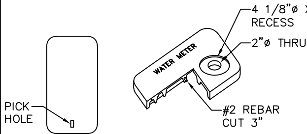
SM30 LID DETAIL
