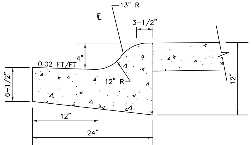
ELEVATION B-B
