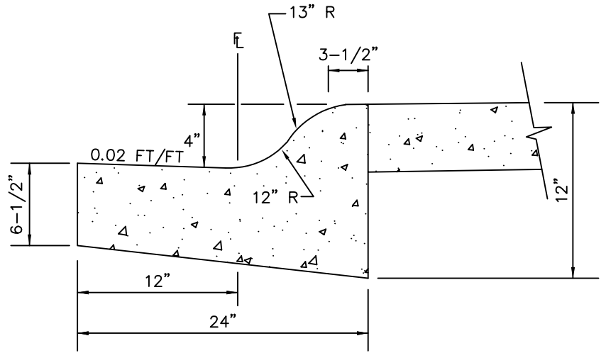
ELEVATION B-B
