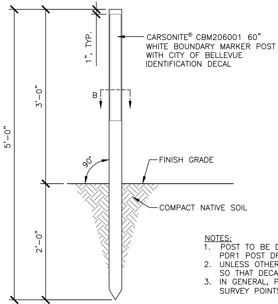
A - ELEVATION
